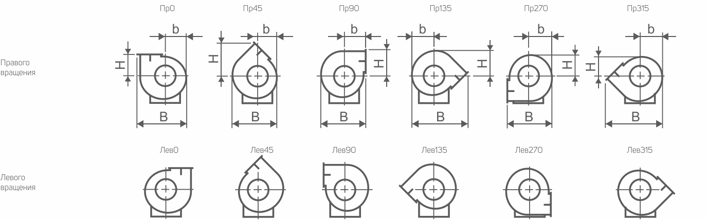
Вид со стороны всасывания
